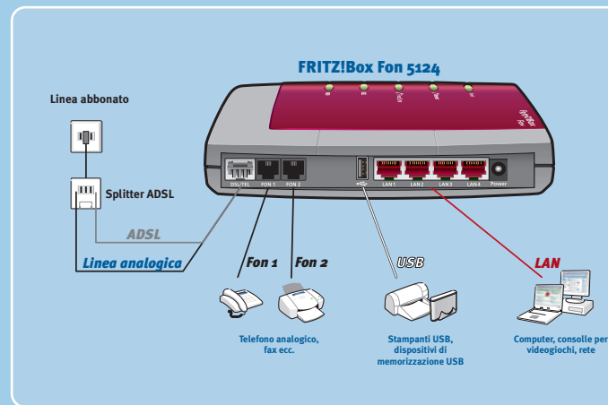
FRITZ!Box Fon 5124 con 1 porta USB e 4 porte LAN; 2 connessioni analogiche
