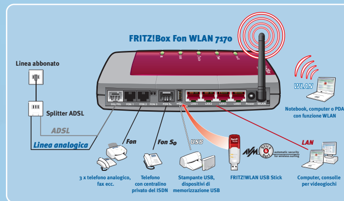
FRITZ!Box Fon WLAN 7170 con 4 porte LAN, 3 connessioni analogiche, S 0 ISDN e una porta per accessori USB
